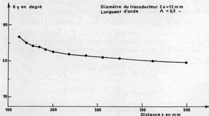
FIG. 11. — \delta\gamma Retard de phase dû à la diffraction suivant un axe binaire du silicium monocristallin.
